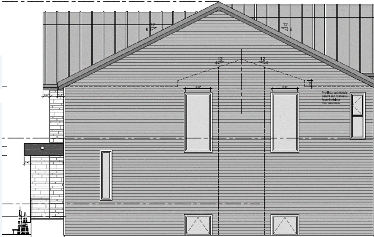
Élévation droite
